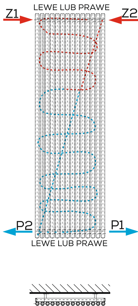
PODŁĄCZENIE KRZYŻOWE
