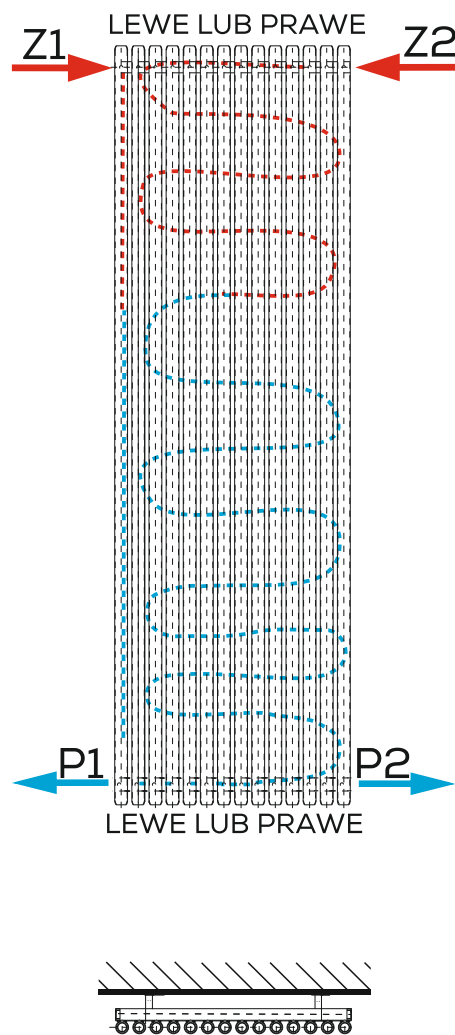
PODŁĄCZENIE STANDARDOWE GÓRA-DÓŁ
