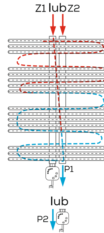
PODŁĄCZENIE KRZYŻOWE
