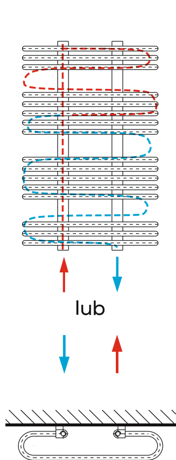
PODŁĄCZENIE OD, DOŁU W KOLEKTORACH
