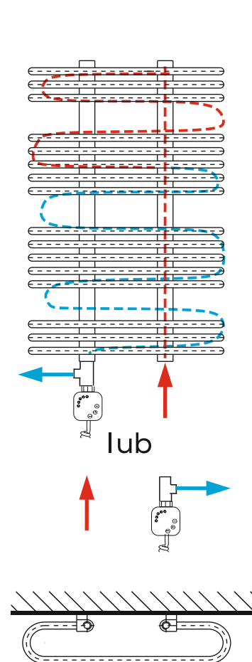
WODNO-ELEKTRYCZNY OD DOŁU W KOLEKTORACH
