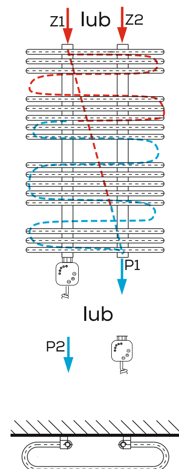
PODŁĄCZENIE KRZYŻOWE
