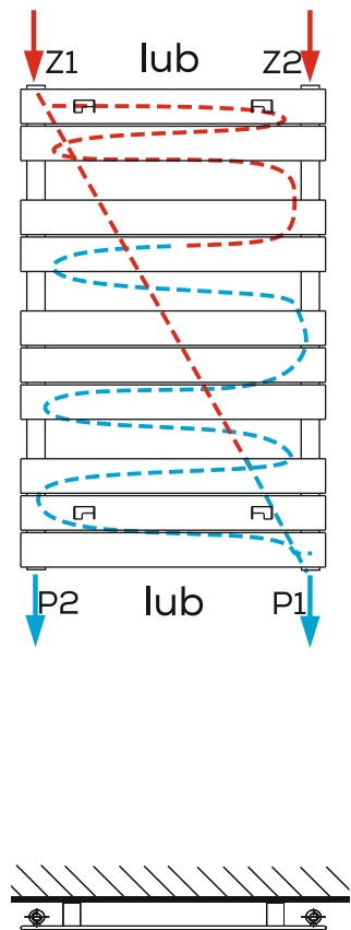
PODŁĄCZENIE KRZYŻOWE
