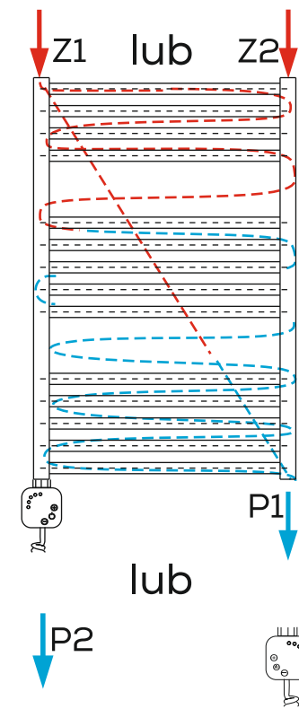
WODNO-ELEKTRYCZNY OD DOŁU W KOLEKTORACH
