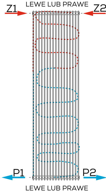
PODŁĄCZENIE STANDARDOWE GÓRA-DÓŁ
