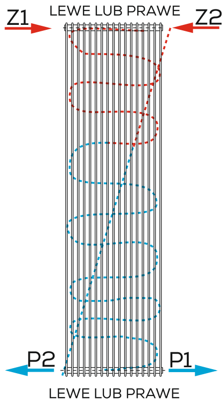
PODŁĄCZENIE KRZYŻOWE
