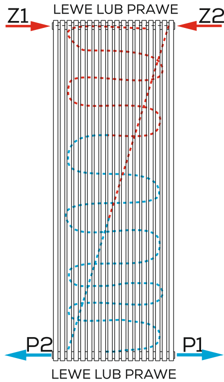
PODŁĄCZENIE KRZYŻOWE
